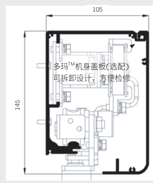
带盖板的运行轨道型材
